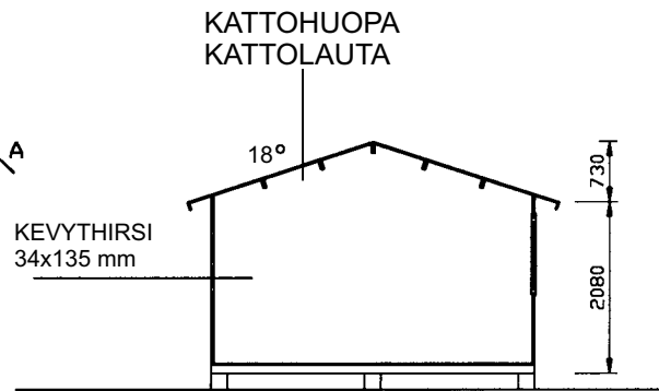
LEIKKAUS A - A
